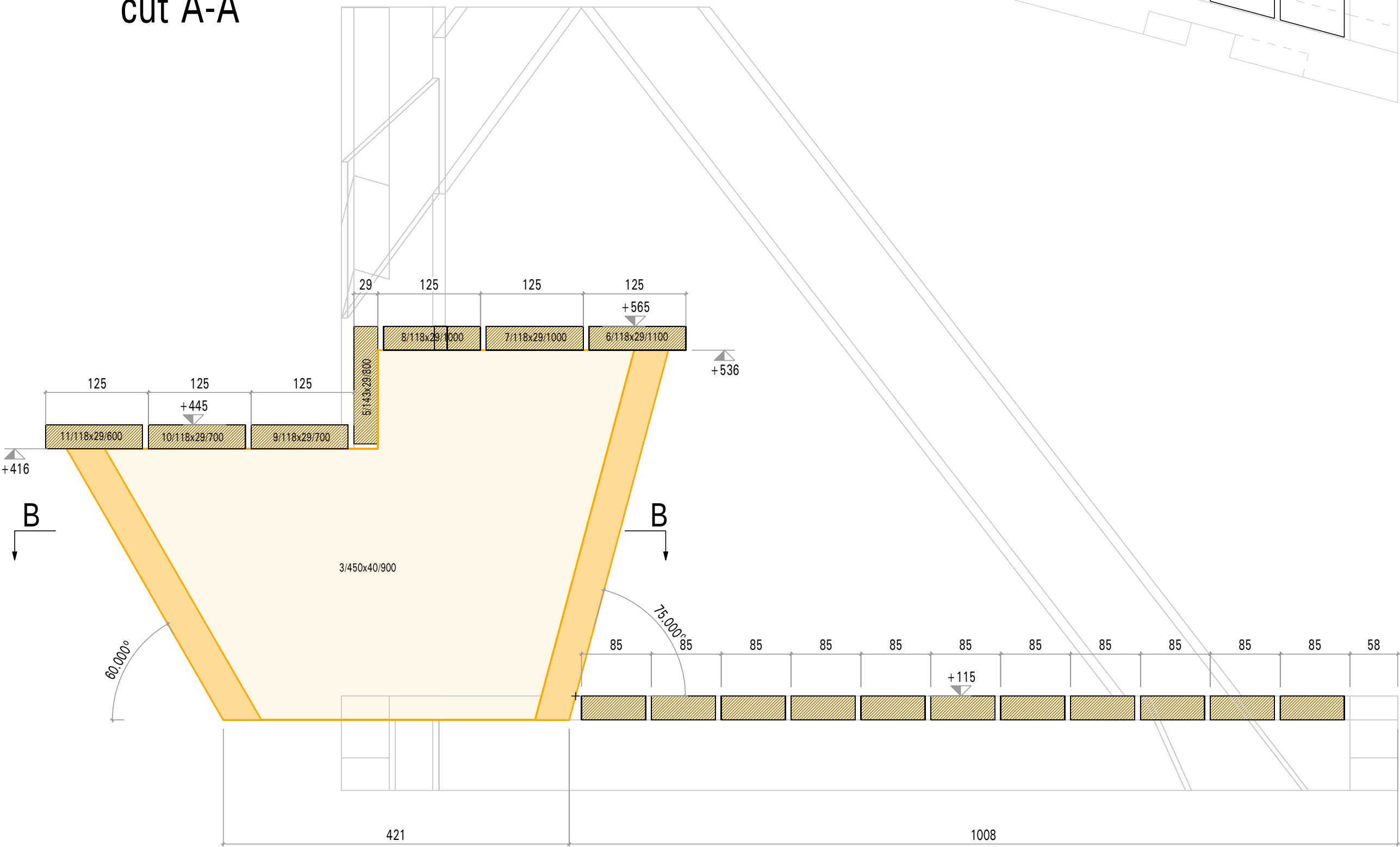
cut A-A
