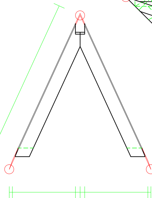
Affasede kvistspær.
